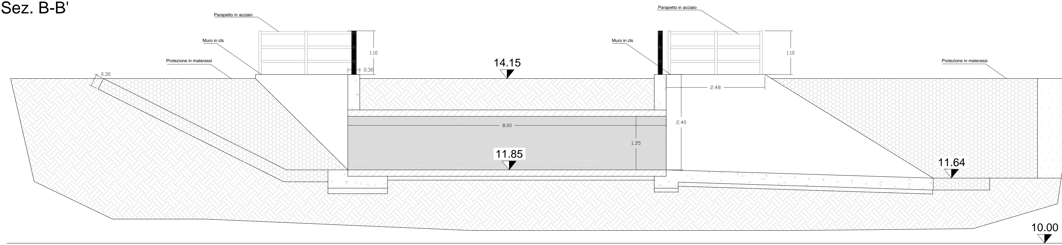
Sez. B-B'
