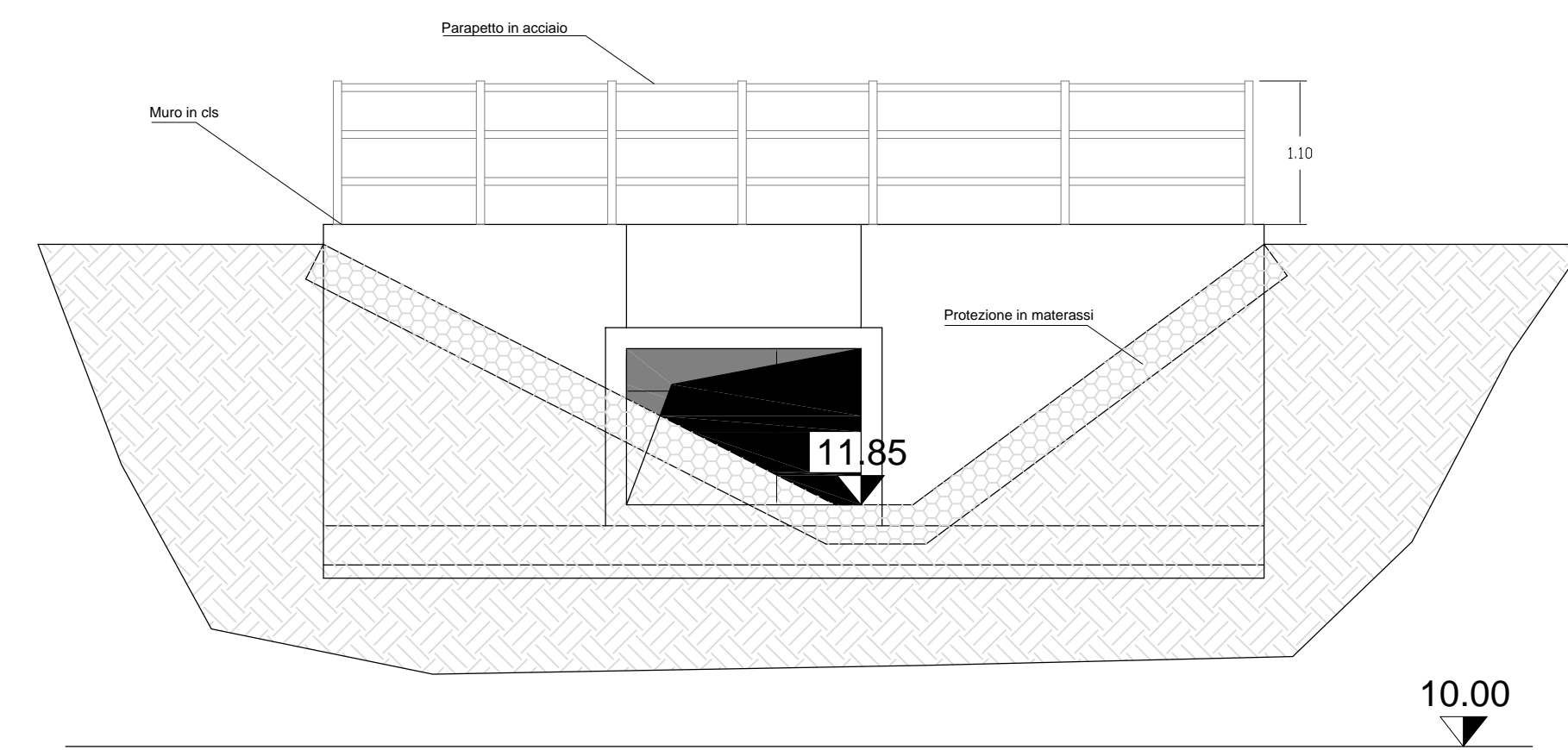
Sez. C-C'
