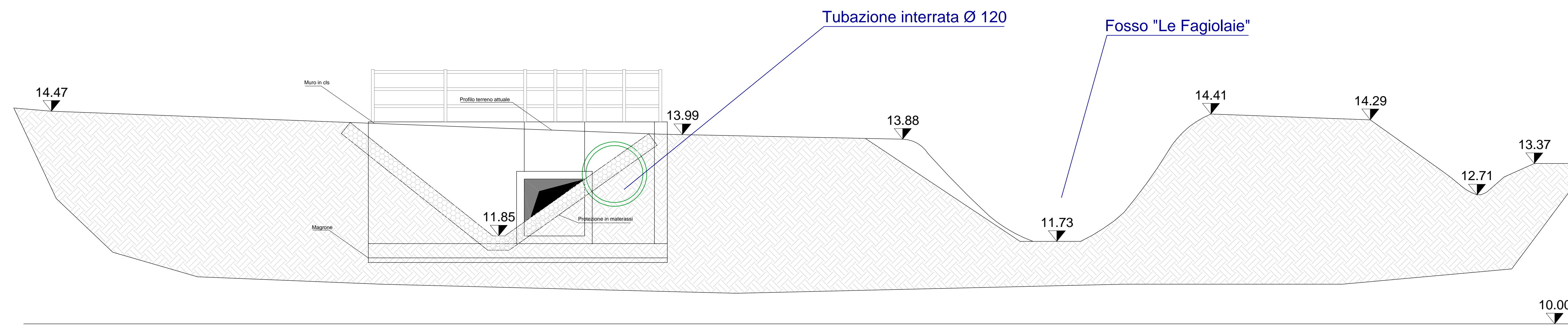
Sez. C-C'
