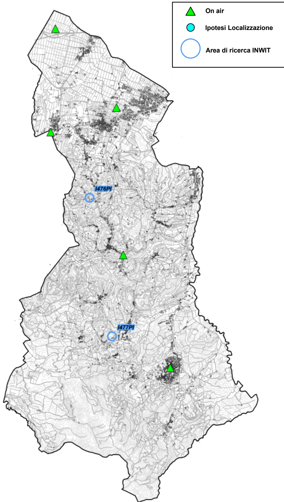
Fig. 21 Piano di rete - Gestore VODAFONE
