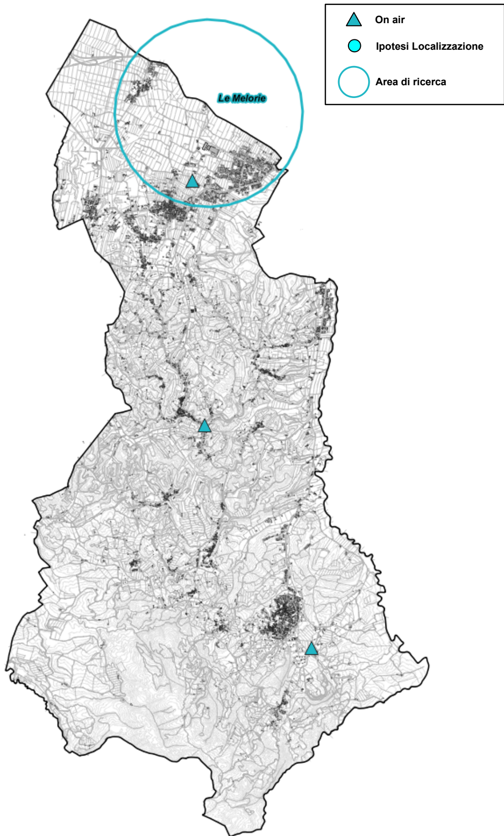
Fig. 25 Piano di rete - Gestore ZEFIRO NET
