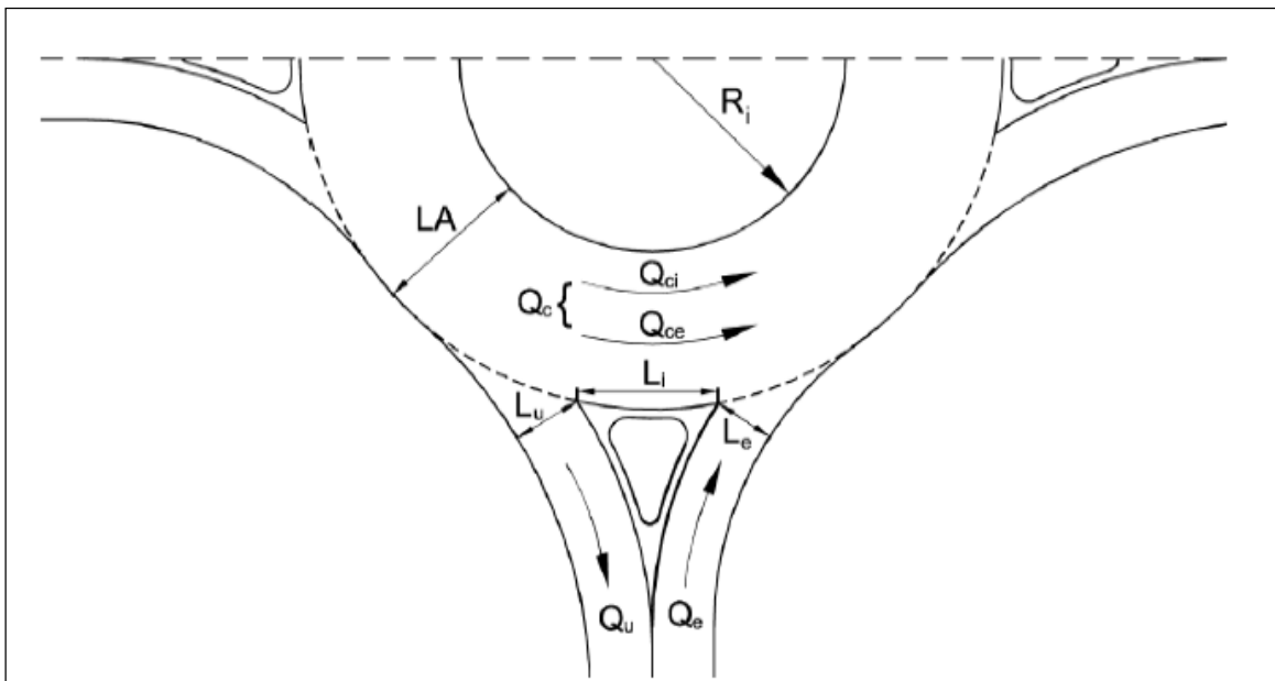
Figura 44 – Grandezze geometriche e funzionali utilizzate dal software Girabase
