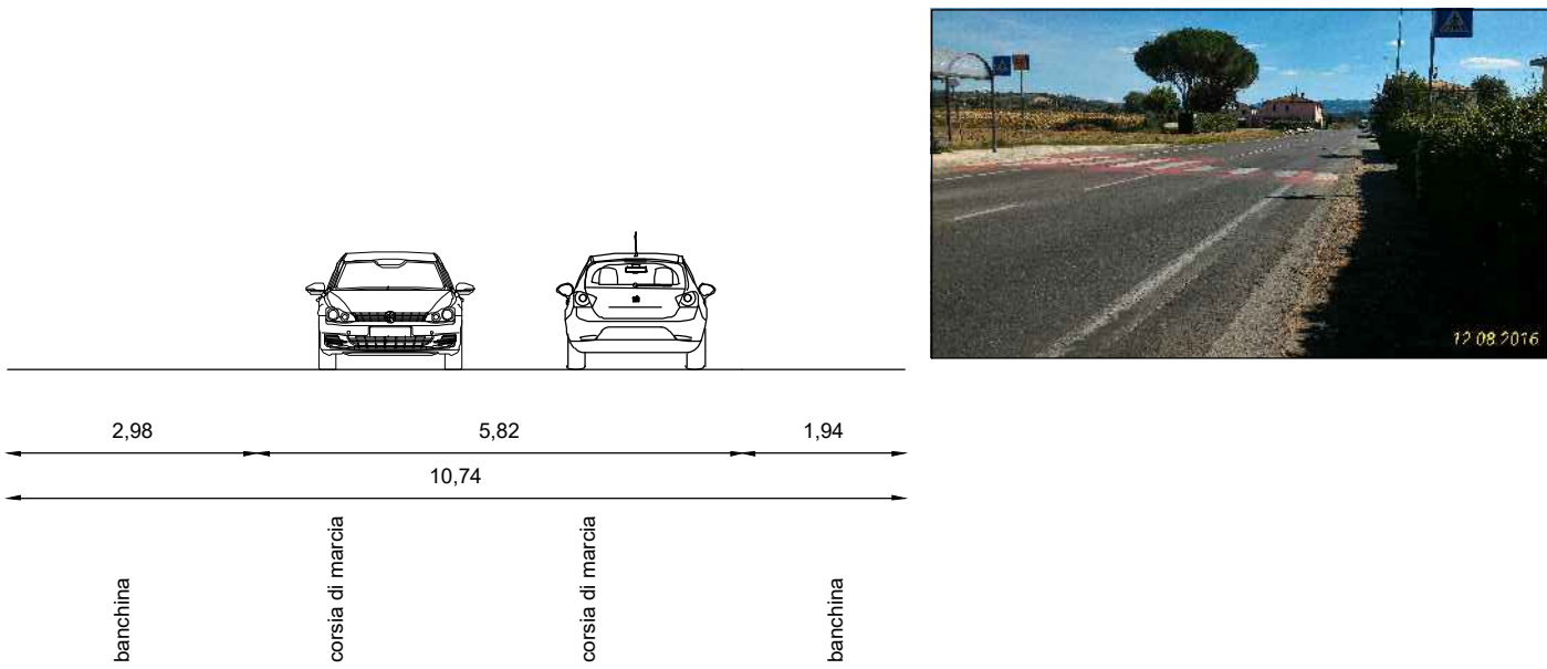
Sezione 100 sp 35
