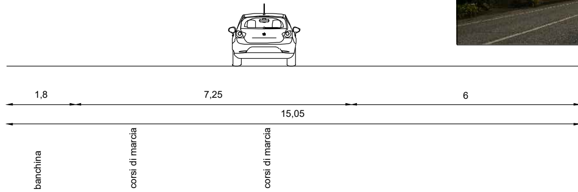
Sezione 5 sp. 12
