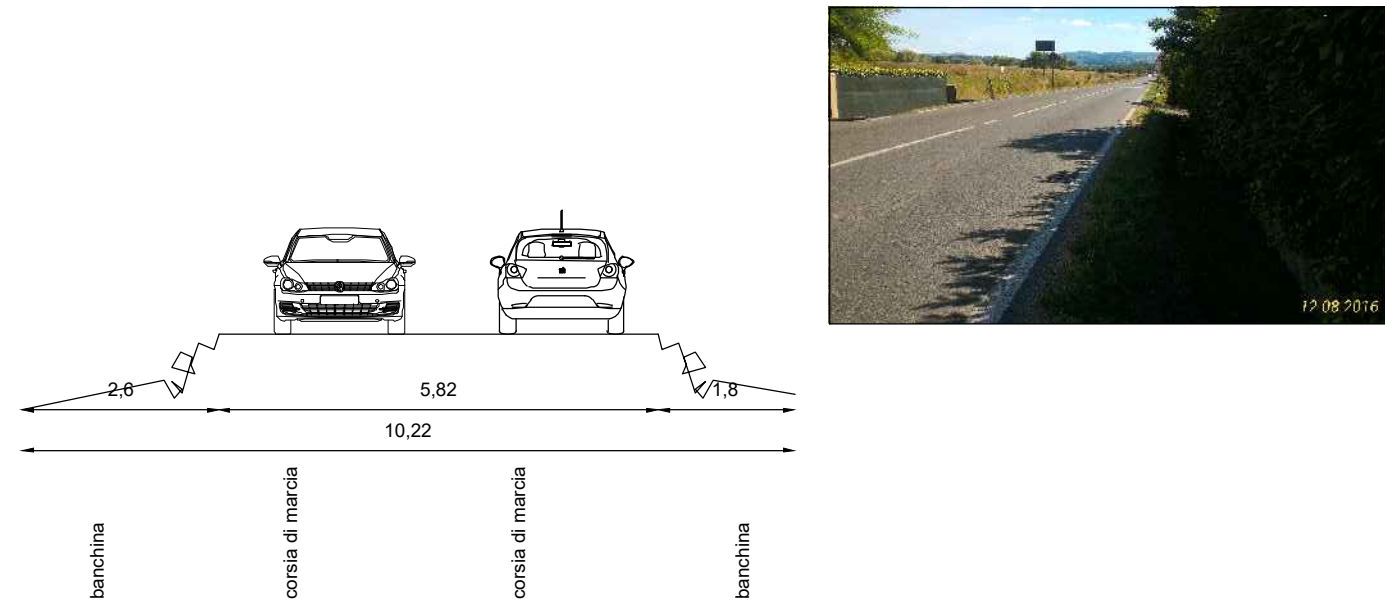
Sezione 101 sp 35
