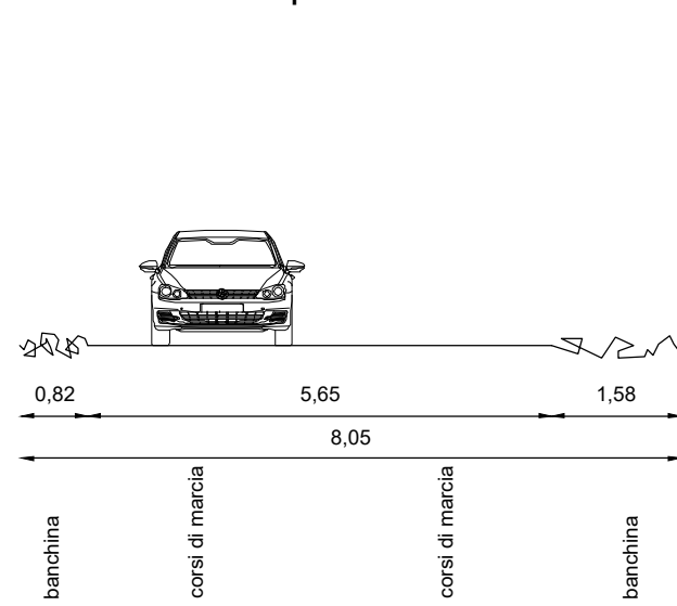
Sezione 64 sp 46
