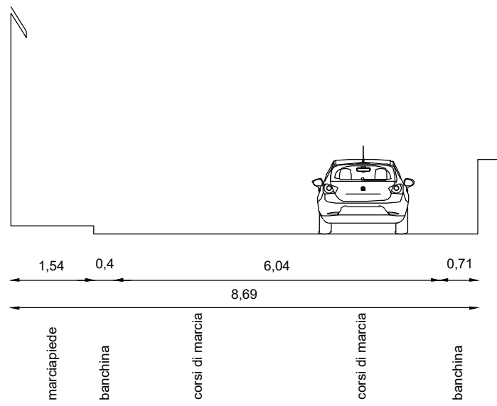
Sezione 62 sp 46
