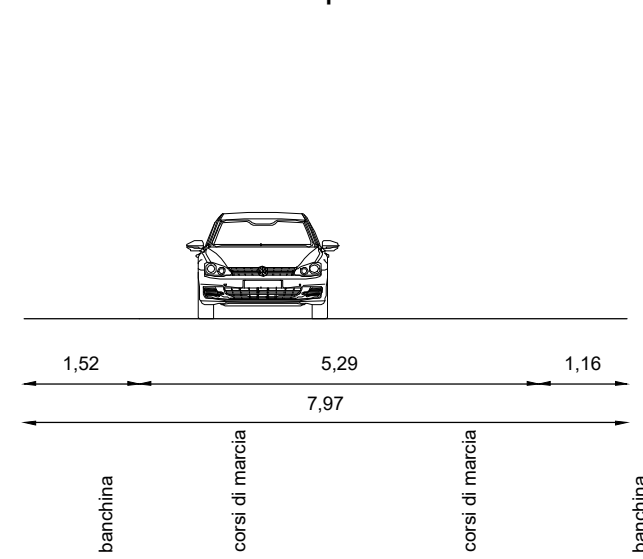
Sezione 65 sp 46
