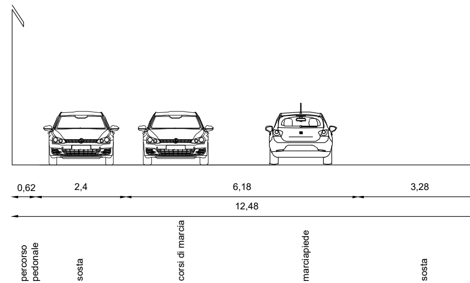
Sezione 53 sp 35
