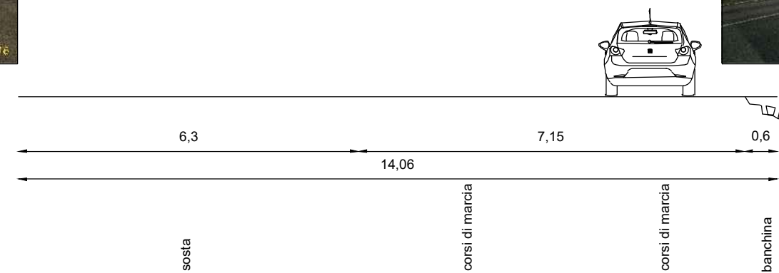
Sezione 6 sp. 12
