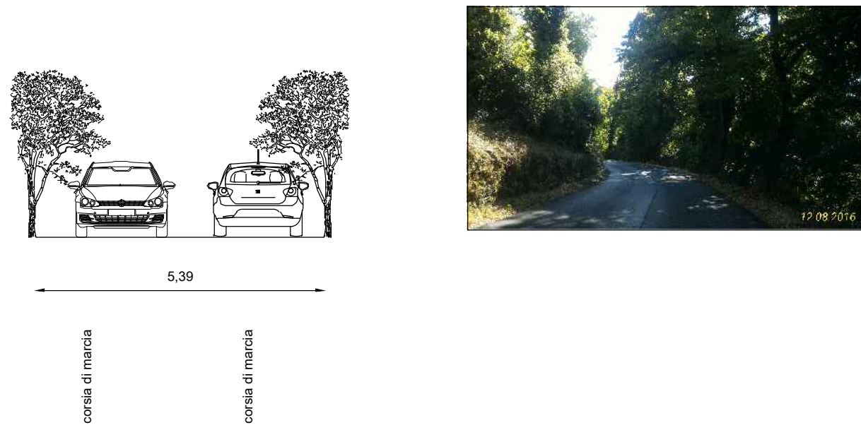
Sezione 100 sp 35
